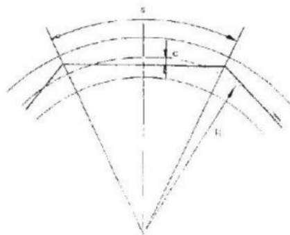
Слика 1: Шематски приказ полигонације Табела 2: Полигонација полукомпензоване контактне мреже
