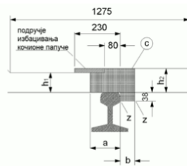
Слика 1: Доњи део слободног профила
