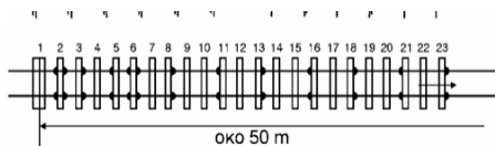
Слика 6: Положај справа против путовања шина за шину типа 49Е1
