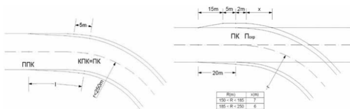
Слика 4: Проширење слободног профила са и без прелазне кривине
