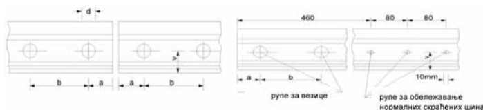
Слика 5: Распоред бушења
