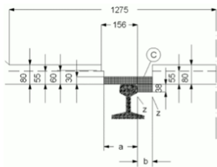
Слика 1: Доњи део слободног профила
