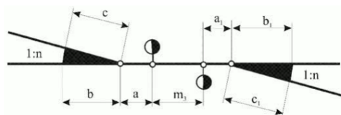
Слика 10: Међуприва између две скретнице са супротно усмерени кривинама
