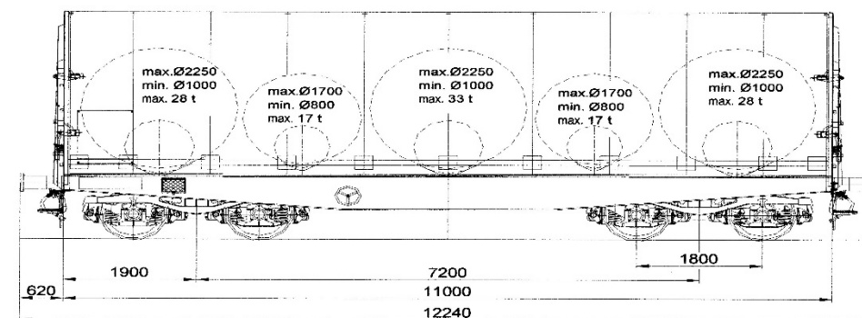
Šema maksimalnog opterećenja kolevki kola serije Shimms
